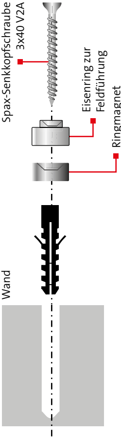
Wandmontage der Wandabreißsicherung
