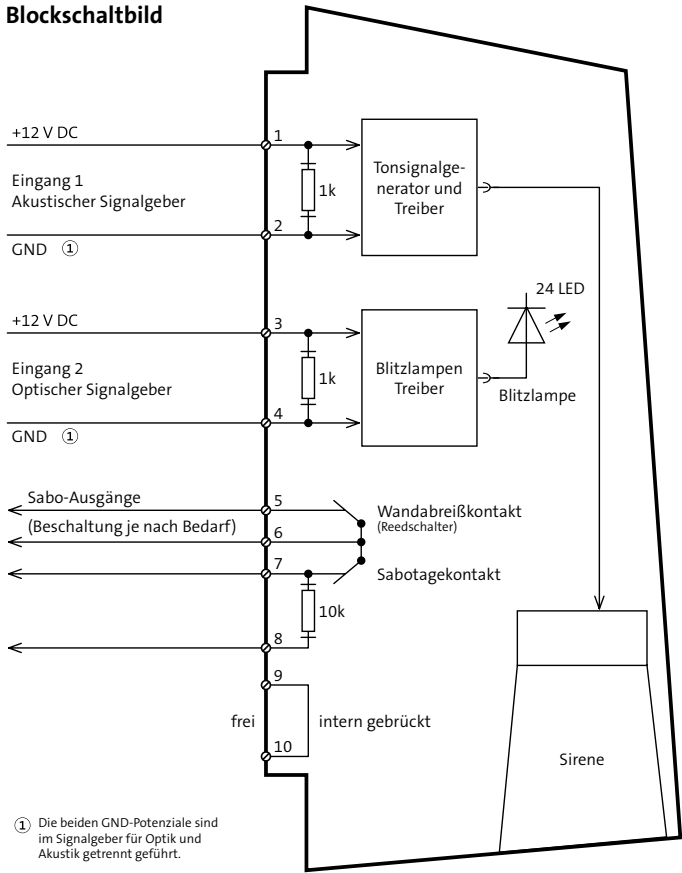
Blockschaltbild
