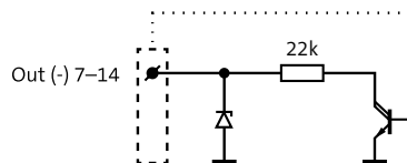
Anschlussplan Out (-) 7–14
