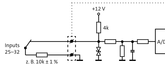
Anschlussplan Inputs 25–32
