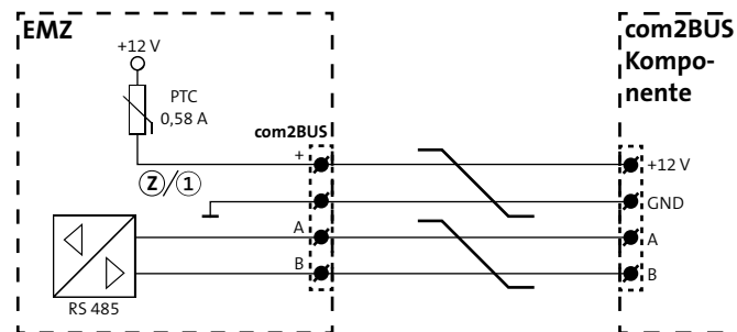
Anschlussschema com2BUS
