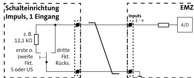
Schalteneinrichtung Impulskontakt, 1 Eingang, 3 Funktionen
