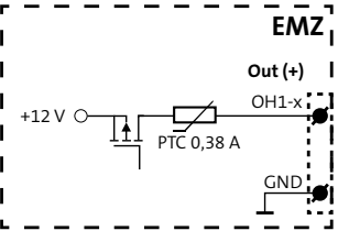
Anschlussschema Spulenausgänge (OH1-2)
