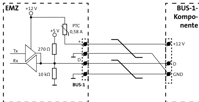
Anschluss BUS-1-Komponente
