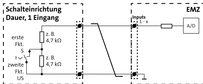
Schaltanlage Dauerkontakt, 1 Eingang, 2 Funktionen
