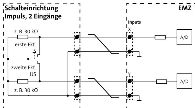
Schaltanlage Impulskontakt, 2 Eingänge, 2 Funktionen
