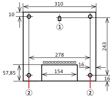
Maßzeichnung Gehäusetyp GR80
