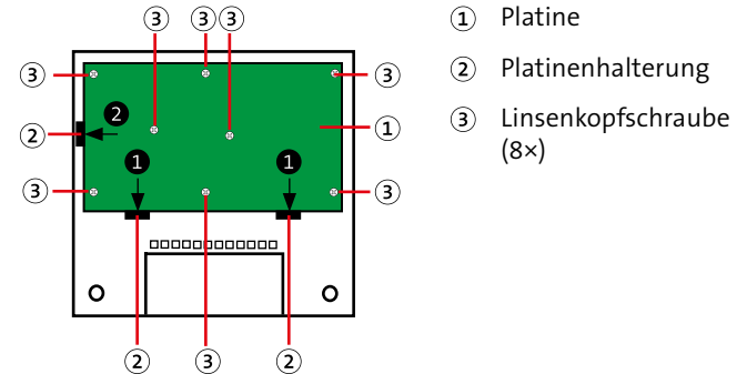
Montage Platine Gehäusetyp GR80
