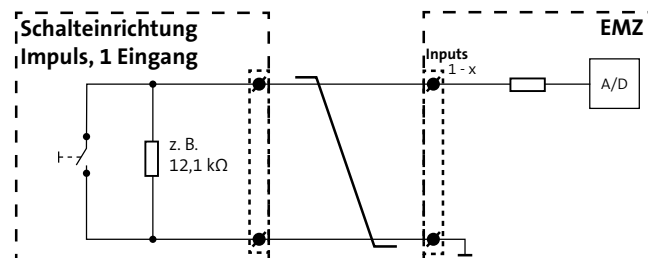
Schteinrichtung Impulskontakt, 1 Eingang, 1 Funktion
