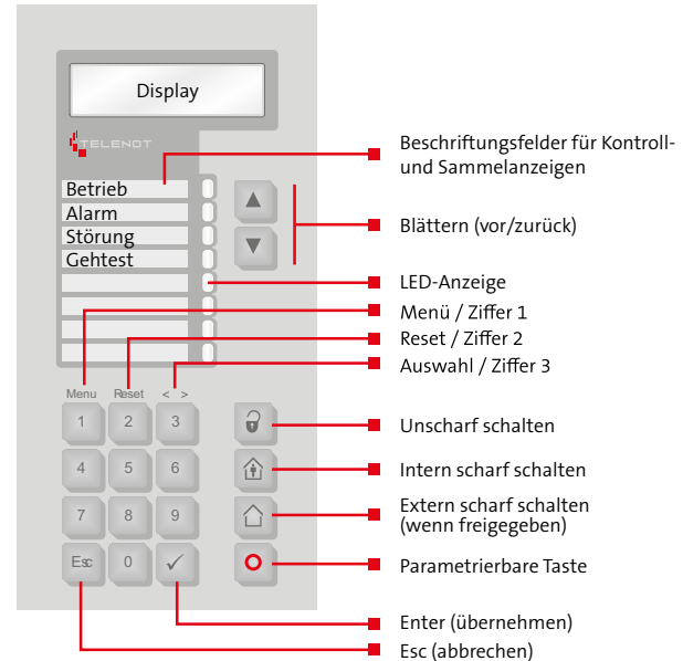
Bedienung BT 820
