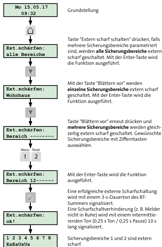
Extern scharf schalten am BT 820
