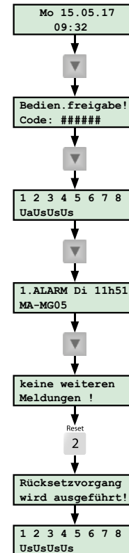
Rücksetzen am BT 820
