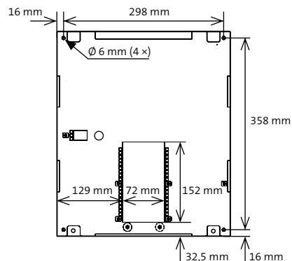
Maßzeichnung Grundplatte Gehäusetyp GR100
