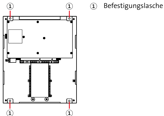
Demontage Rahmen Gehäusetyp GR100
