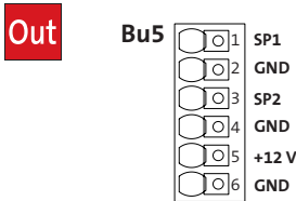
Anschlussbelegung SP1/SP2 und 12-V-Versorgung (Bu5)
