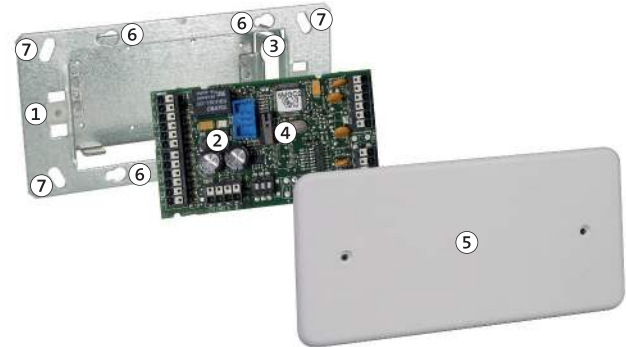
Mechanischer Aufbau 5-MGM C2B uP für Unterputzmontage
