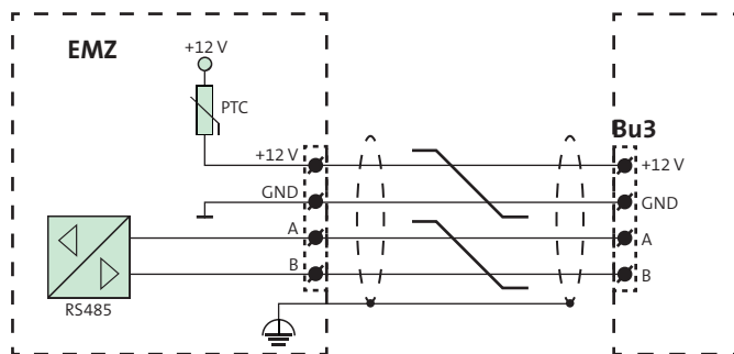
Anschlussschema com2BUS
