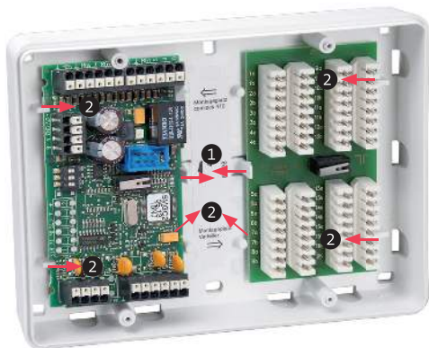
Beispiel Demontage der Platinen im Gehäusotyp K30
