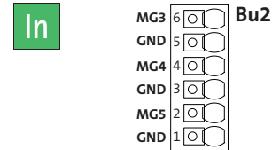
Anschlussbelegung Meldergruppen (In) MG3 bis MG5 (Bu2)
