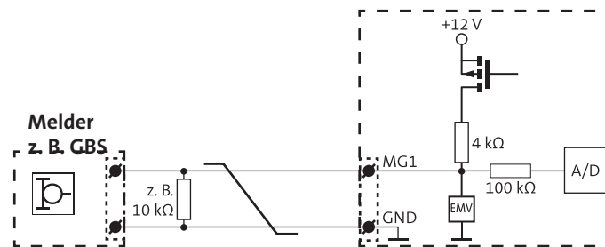
Anschlussschema MG1
