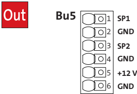
Anschlussbelegung SP1/SP2 und 12-V-Versorgung (Bu5)
