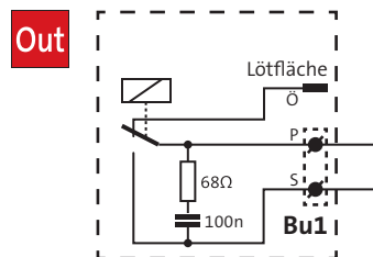
Anschlusschema Relaisausgang
