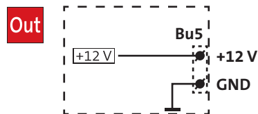
Anschlusschema +12-V-Versorgungsspannung
