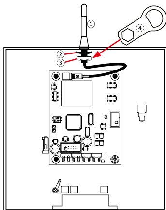
Montage der Antenne auf das GR10-Gehäuse
