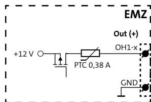
Anschlussschema Spulenausgänge (OH1-4)
