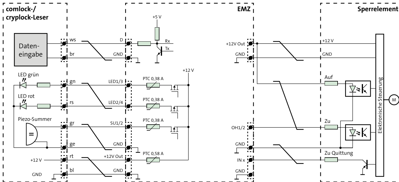
Anschlussschema comlock-/cryptlock-Leser (Reader 1/2)
