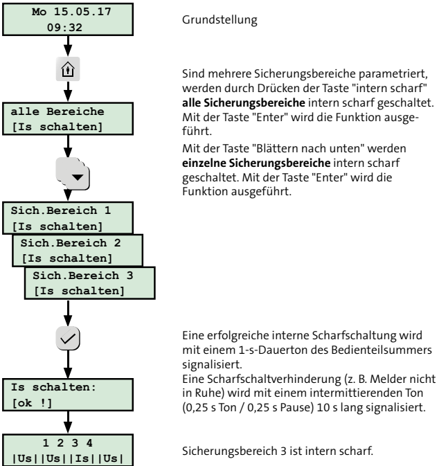
Abb.: Intern scharf schalten mit Bedienteil
