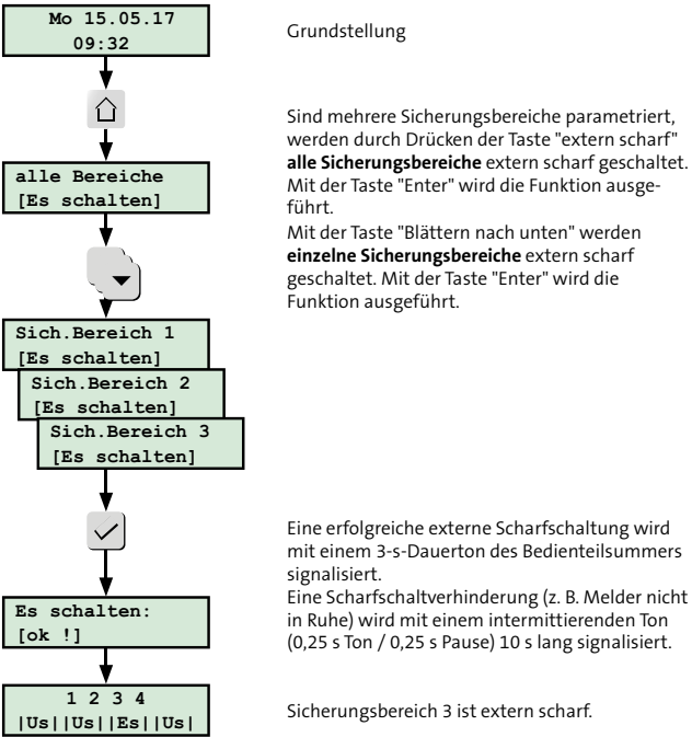
Abb.: Extern scharf schalten mit Bedienteil
