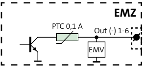
Anschlusschema Transistorausgänge 1-6 Out (-)
