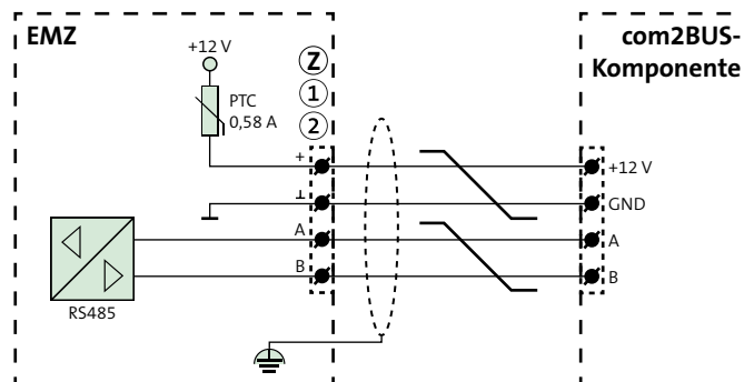
Anschlusschema com2BUS
