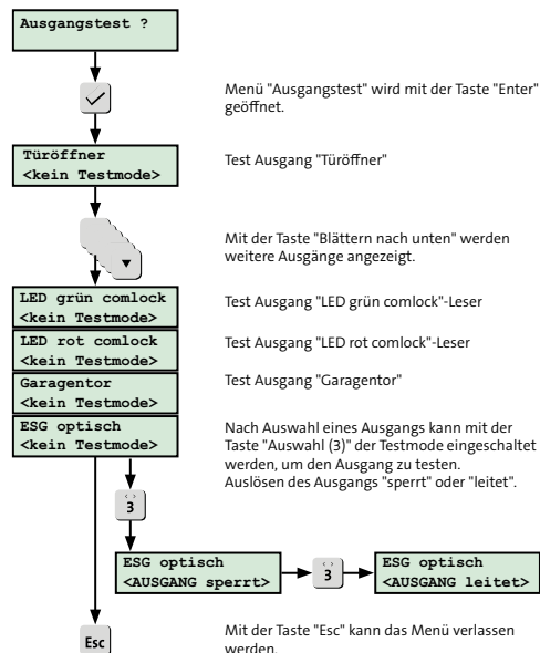
Abb.: Menü Ausgangstest
