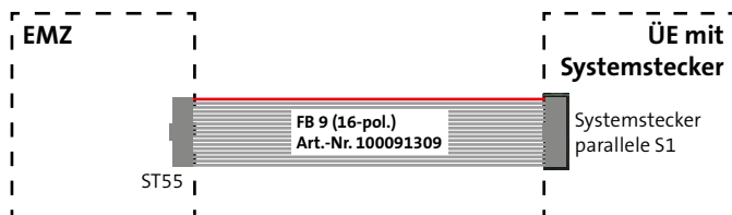
Anschlussschema eingebaute ÜE mit Systemstecker
