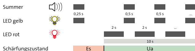
Abb.: Unscharf schalten mit Transponder am cryclock-Leser
