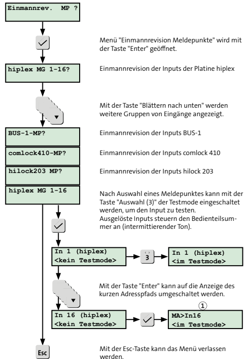
Abb.: Menü Einmannrevision Meldepunkte
