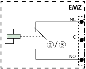
Anschlusschema Relaisausgänge REL 2-3
