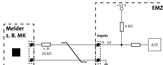
Anschlusschema Inputs 9-16
