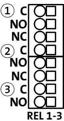
Abb.: Anschlussbelegung REL 1-3
