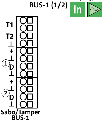
Abb.: Anschlussbelegung Deckelkontakt, Abreißmelder und BUS-1 (1/2)
