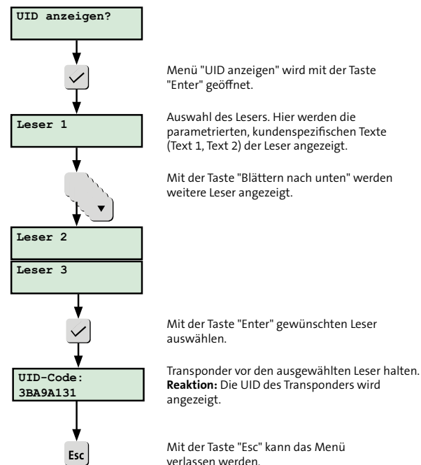
Abb.: Menü UID anzeigen
