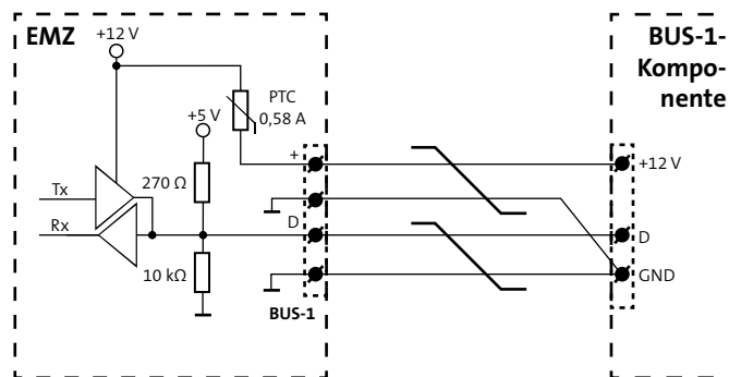
Abb.: Anschluss BUS-1-Komponente
