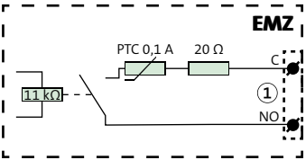
Anschlusschema Relaisausgang REL 1
