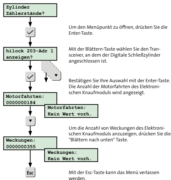
Abb.: Menü Zylinder Zählerstände
