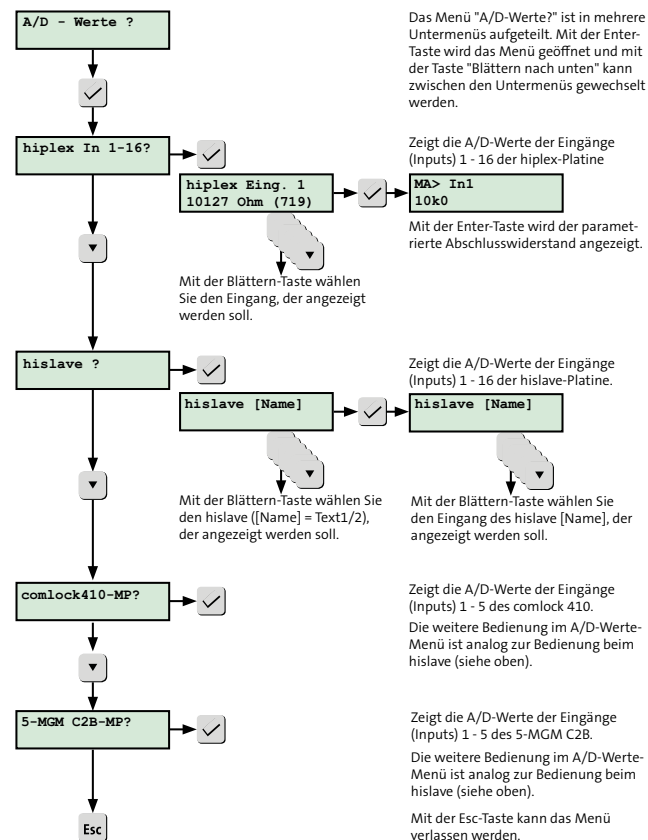
Abb.: Menü A/D-Werte
