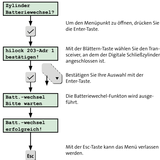
Abb.: Menü Zylinder Batteriewechsel
