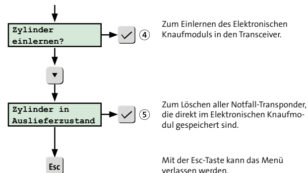
Abb.: Menü Zylinder DSZEK
