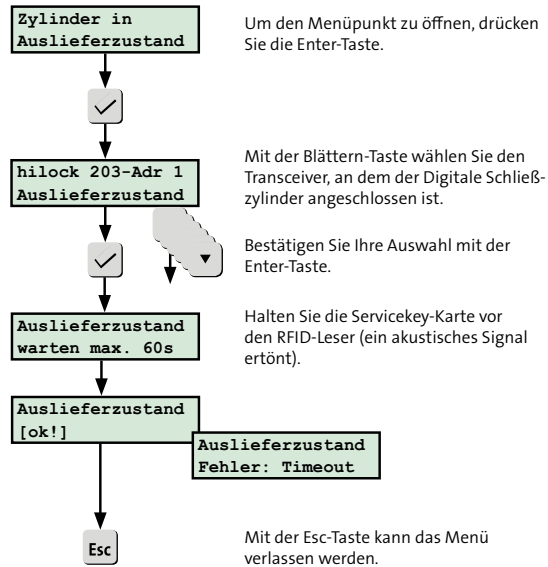
Abb.: Menü Zylinder Auslieferungszustand
