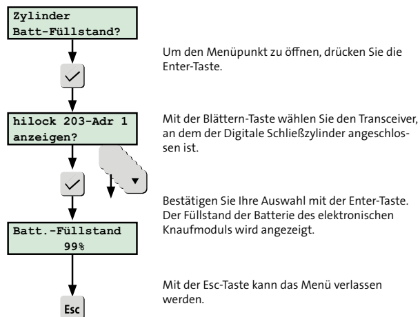
Abb.: Menü Zylinder Batterie-Füllstand
