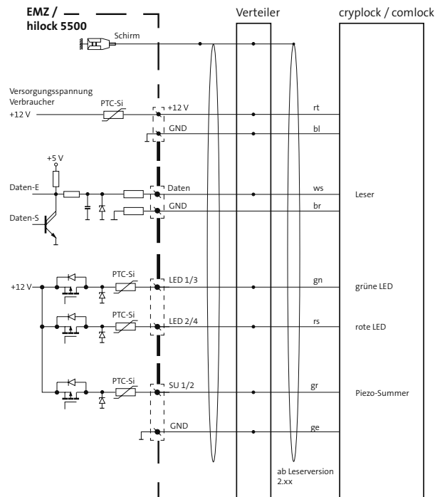
Anschaltplan Leser an EMZ / hilock 5500
