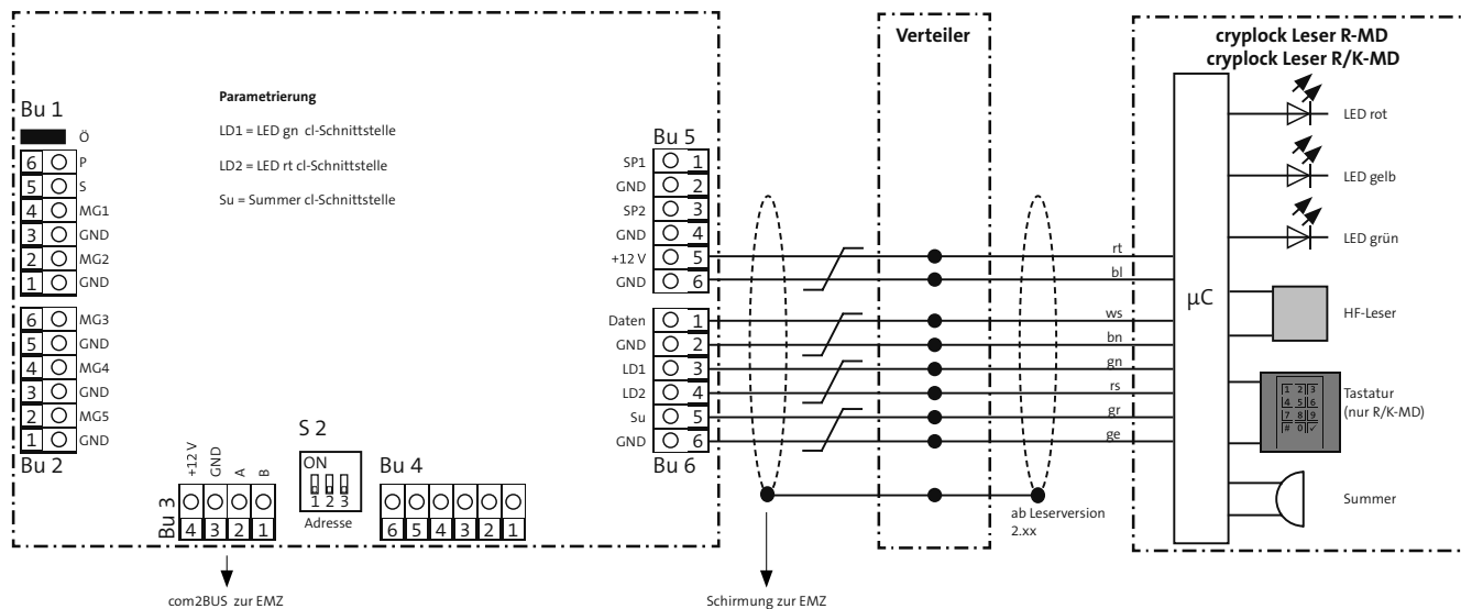
Anschaltplan Leser am Türmodul
