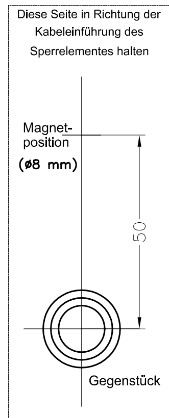
Abbildung 5-2 Bohrschablone Magnetposition im Türblatt
