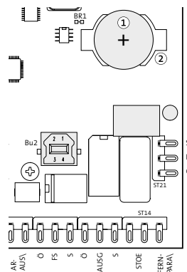
Einsetzen der Lithium-Knopfzelle
