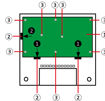
Montage Platine Gehäusotyp GR80
